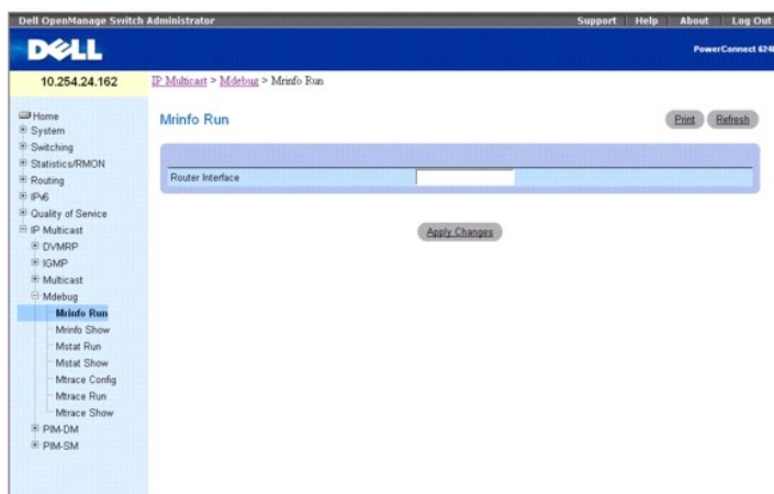
Рис. 12-23. Запуск MRinfo
