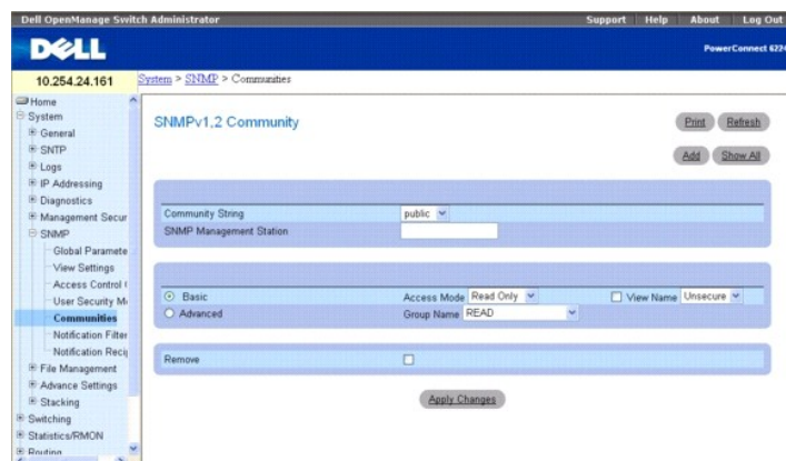
Рис. 6-63. SNMPv1, 2 Сообщество
