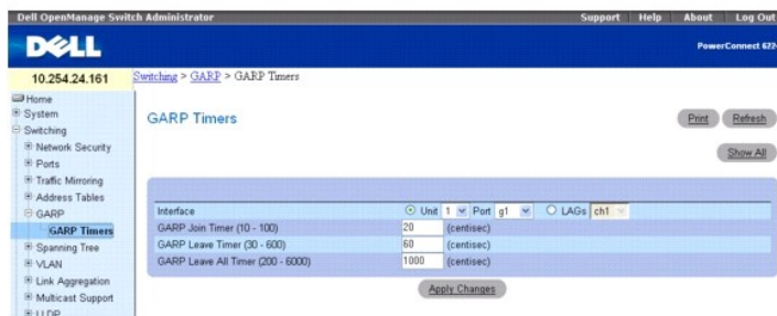
Рис. 7-33. Таймеры GARP
