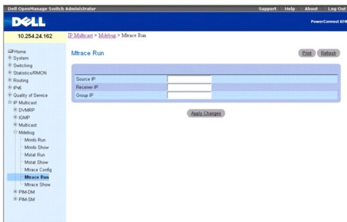
Рис. 12-28. Запуск MTrace
