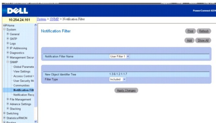
Рис. 6-66. Фильтр извещений
