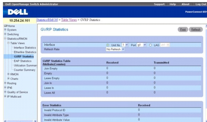
Рисунок 8-3. Статистика GVRP
