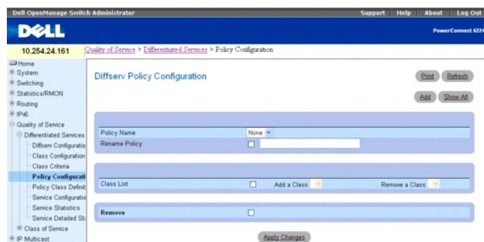
Рисунок 11-6. Конфигурация политики
