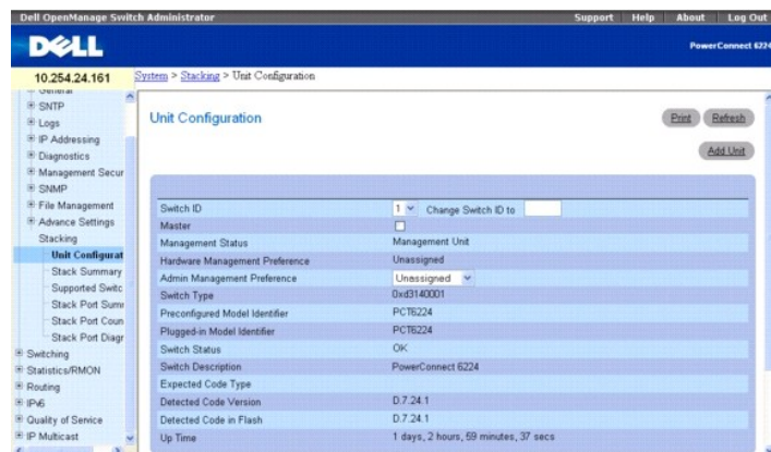
Рис. 6-78. Конфигурация устройства
