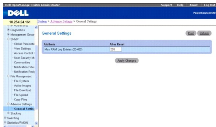
Рис. 6-77. Общие параметры
